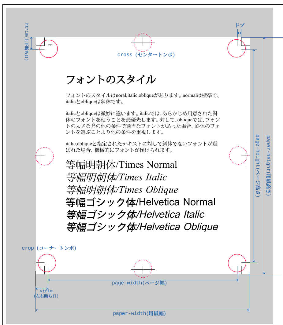
図 4.20 ページのレイアウト
